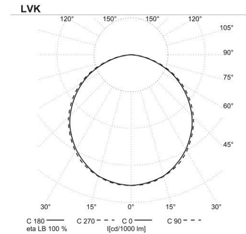
Lichtverteilungskurve
