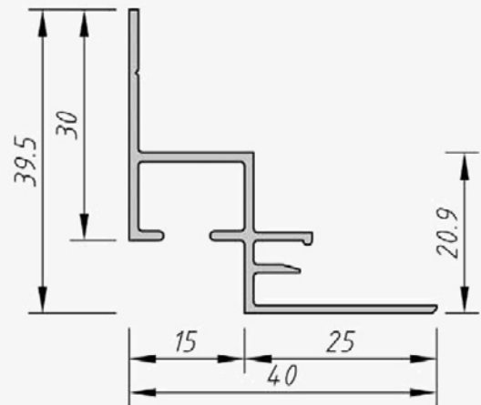
Bilderschiene 15/10
