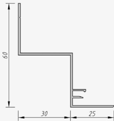
Schattenfederleiste 30/30
