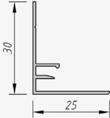
Federleiste 30/25
