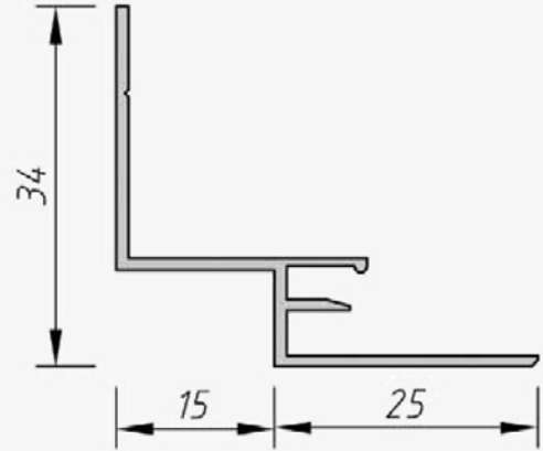
Schattenfederleiste 15/10
