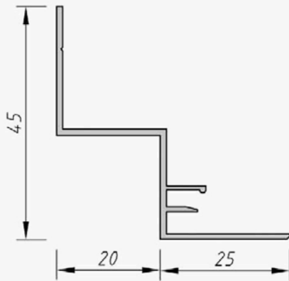
Schattenfederleiste 20/20
