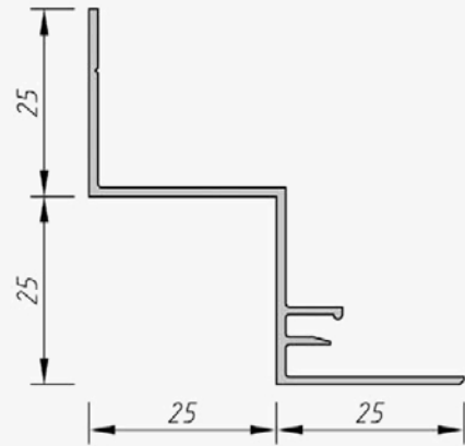
Schattenfederleiste 25/25
